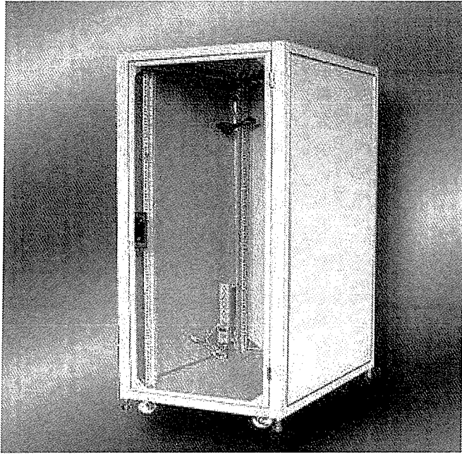
外部尺寸：寬：60cm / 高：約 109cm(含輪子) / 深：100cm
