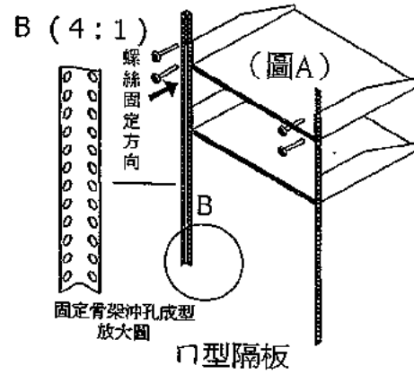
內層格板固定示意圖
