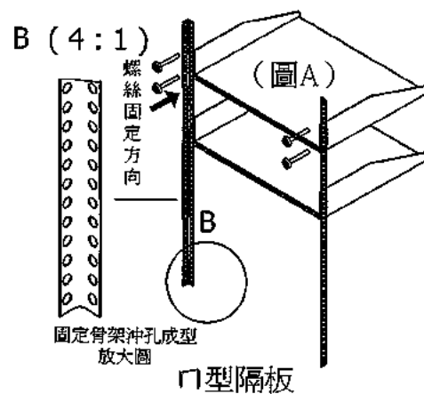
內層格板固定示意圖
